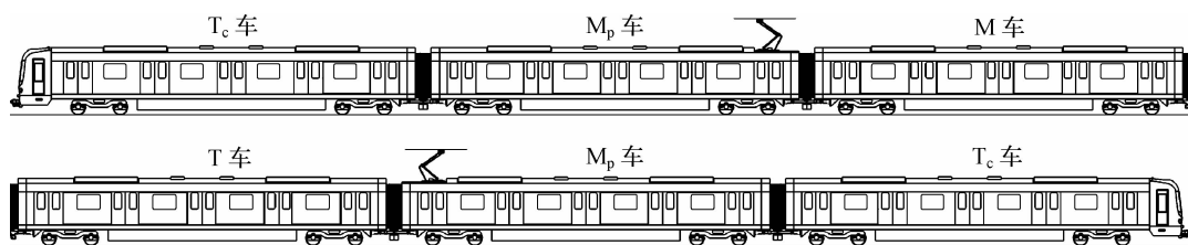
图 1-13 某地铁 2 号线车辆的编组情况
