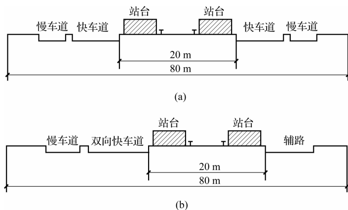
图 1-5 地面线路设置
