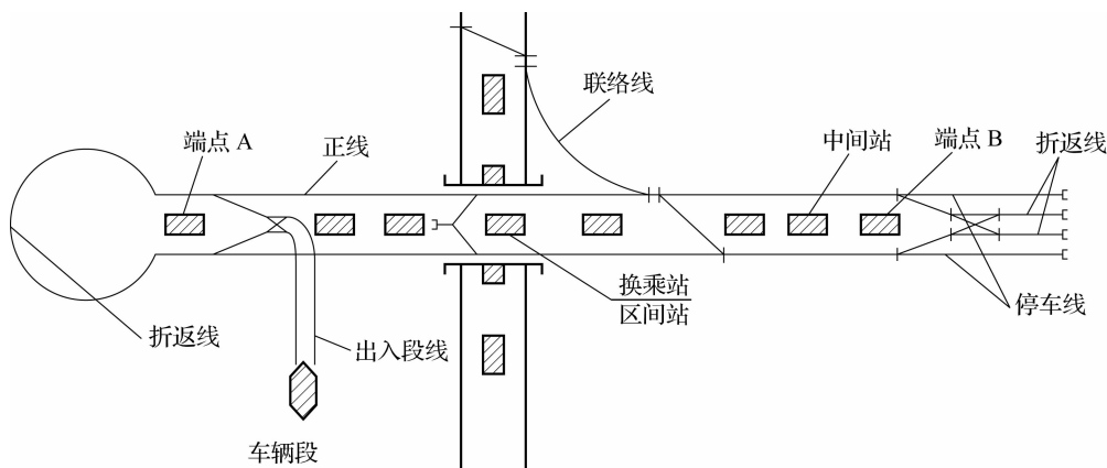
图 1-7 城市轨道交通线路的整体布置
