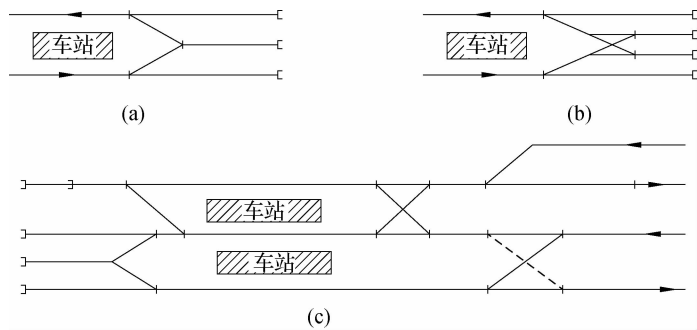
图 1-8 尽端折返线
