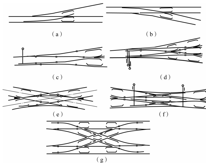
图 1-1 道岔的类型
