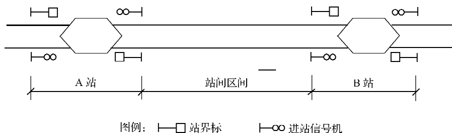
图 1-25 双线线路区间的划分
