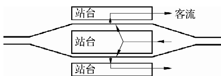
图 1-22 混合式车站
