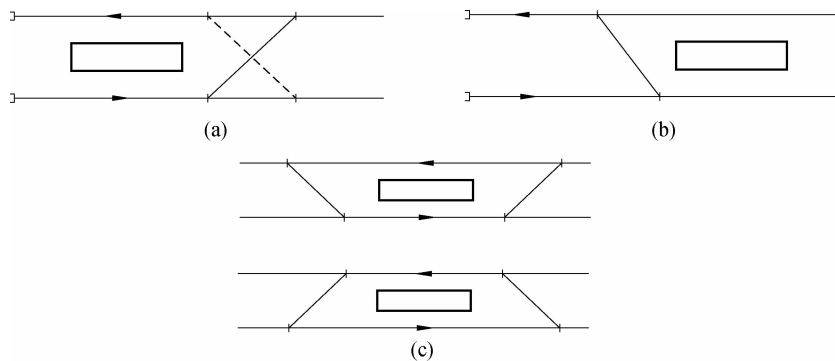
图 1-11 渡线折返线
