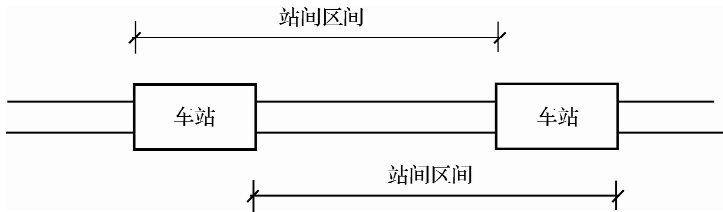
图 1-28 站间区间的划分
