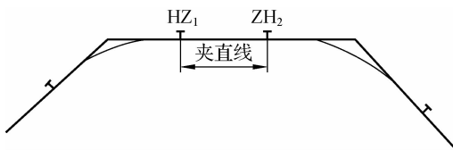
图 1-13 同向曲线
