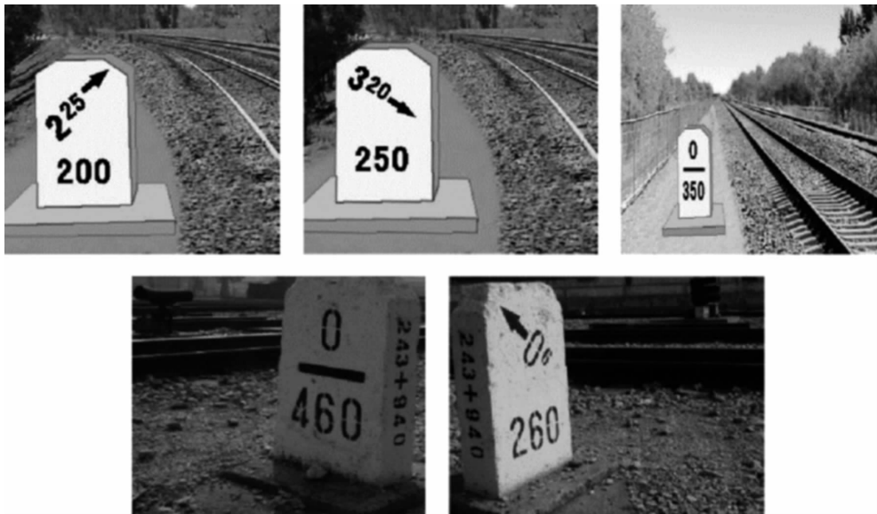
图 1-9 坡度标
