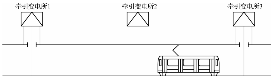
图 1-18 大双边供电
