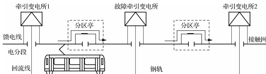
图 1-16 越区供电
