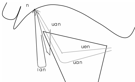
图 1-12 鼻韵母舌位示意(2)
