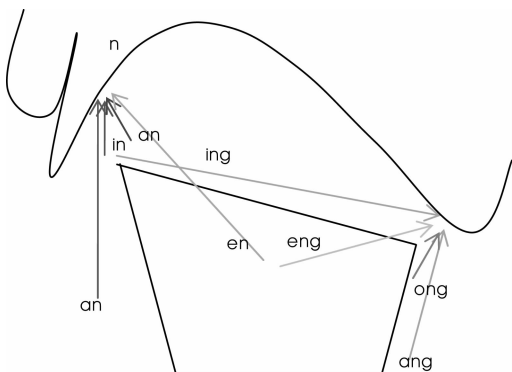
图 1-11 鼻韵母舌位示意(1)
