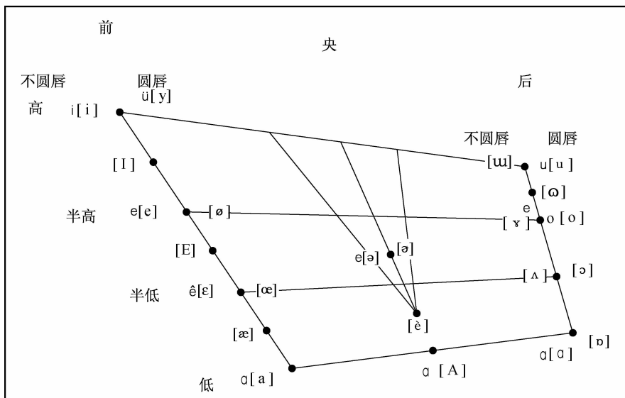
图 1-8 单韵母的舌位示意 (单韵母 a、o、ê、e、i、u、ü、er 的舌位示意)
