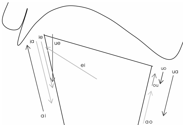
图 1-9 复韵母的舌位示意 (复韵母 ai、ia、ie、üe、ei、ao、ou、uo、ua 的舌位示意)
