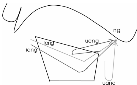
图 1-13 鼻韵母发音示意(3)
